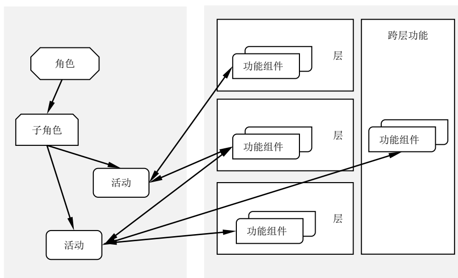
图6 从用户视图到功能视图
